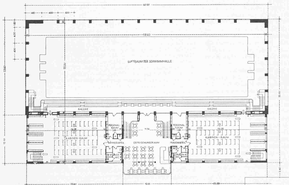
Abb. 10. Obergeschoss mit dem Erfrischungsraum und den oberen Kabinenräumen. — 1:500
