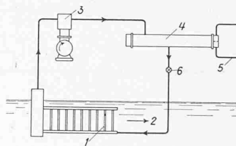
Abb. 21. Berieselungsverdampfer
