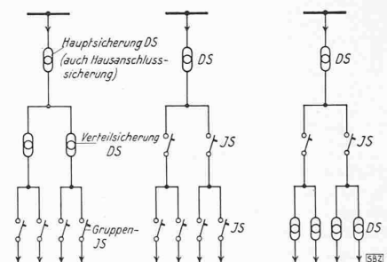
Abb. 5/7. IS als Verteil- u. Gruppensicherung
