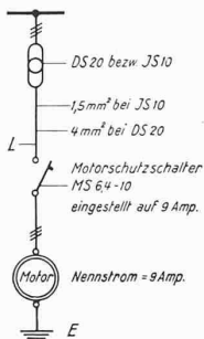
Abb. 8. Schema zu
