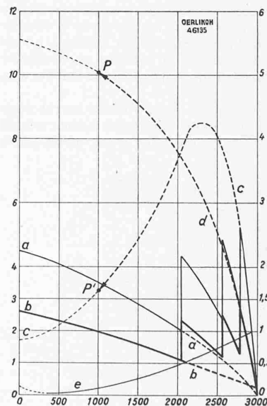
Abb. 2. Anlaufdiagramm eines zweipoligen Combi-Motors beim Antrieb einer Zentrifugalpumpe. Legende: a Drehmoment; b Anfahrstrom bei offener Wicklung II; c Drehmoment; d Anfahrstrom bei kurzgeschlossener Wicklung II; e Lastmoment; P, P' Strom und Drehmoment bei Rückfahldrehzahl des Kontaktes K_3 . — resultierender Anlaufstrom, — resultierendes Anfahrmoment.
