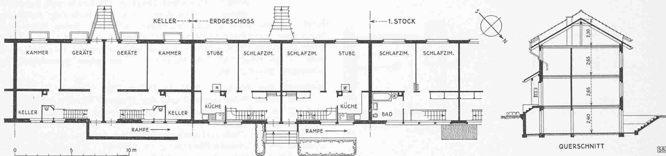
Abb. 9. Siedlung der Schweiz. Draht- und Gummiwerke in Altdorf (Uri). — Entwurf Arch. HERMANN MEYER, Zürich-Oerlikon. — 1:300
