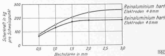
Abb. 6. Einfluss des Elektroden- \varnothing auf die Scherfestigkeit
