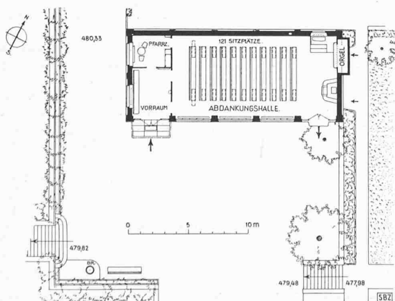
Abb. 13. Abdankungshalle, Grundriss 1:400
