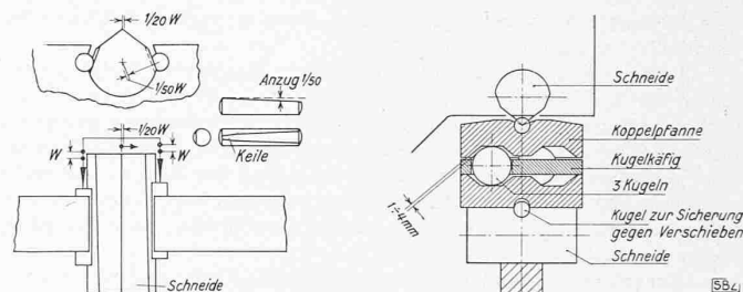
Abb. 9. Schneide mit Zylindersitz
