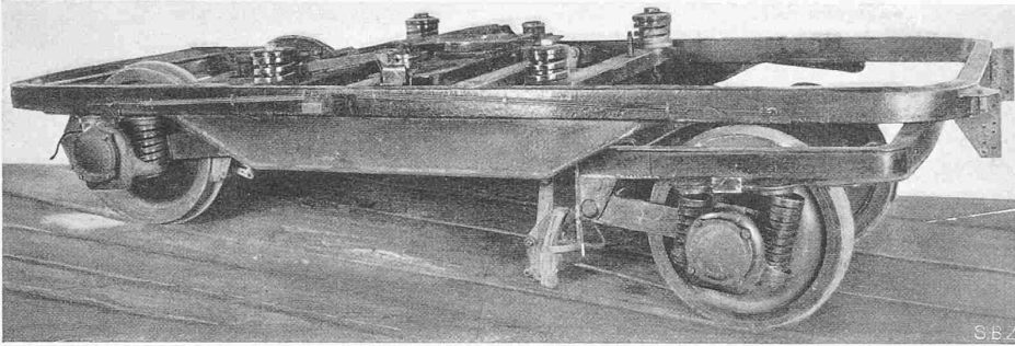
Abb. 3. Drehgestell mit Hohlrahmen und gelenkten Achsen, Radstand 3500 mm
