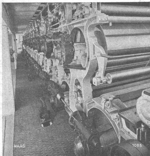
Antrieb von Trockenzyklindern in schweizerischer Papierfabrik mittels Maag-Schneckengetrieben. Insgesamt 26 Getriebe geliefert für diese Anlage.
