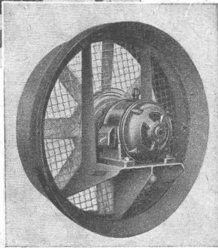
Siemens-Betz-Schraubenlüfter
