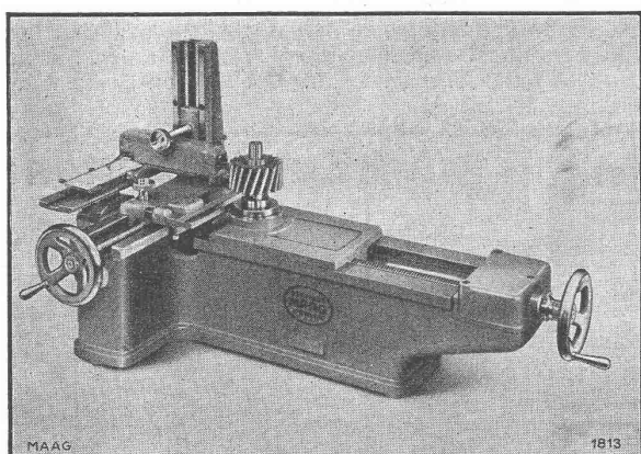
MAAG-Flankenprüfgerät, Typ FPV-40, zur Kontrolle des Zahnprofils an Stirn- und Schraubenrädern.
