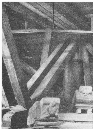
Abb. 6 u. 7. Alter Zustand (Hilfssprengwerke über altem Saal, vergl. Abb. 1 und 2)
