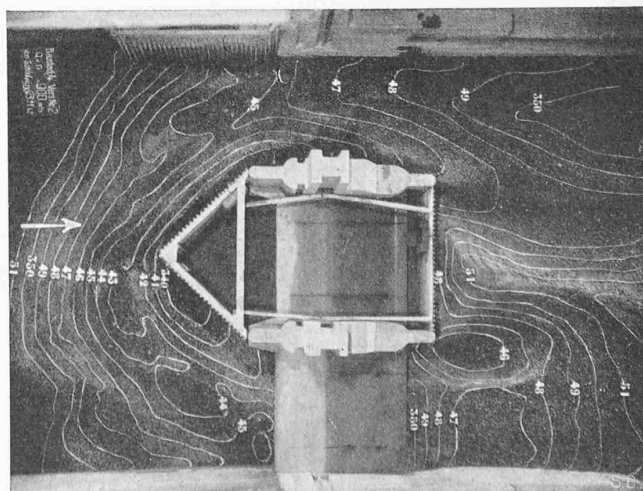
Abb. 4. Baustadium 4 (900 m³/s)
