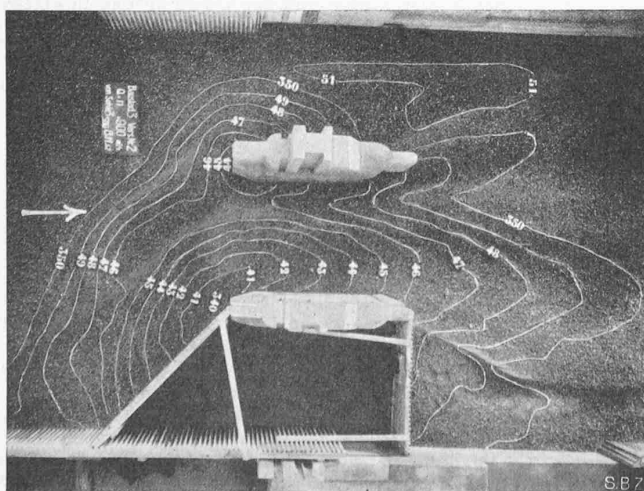
Abb. 3. Baustadium 3 (900 m³/s)
