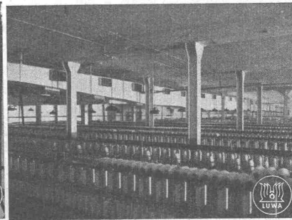
Klimatisierter Ringspinnsaal in einer Gross-Spinnerei
