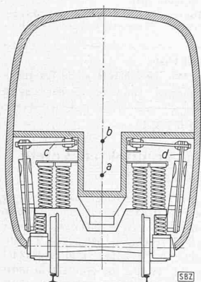
Abb. 1. Schema der Aufhängung
