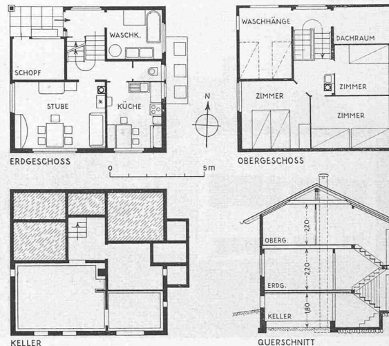
Abb. 5. Grundrisse und Schnitt 1:250 vom kleineren Typ
