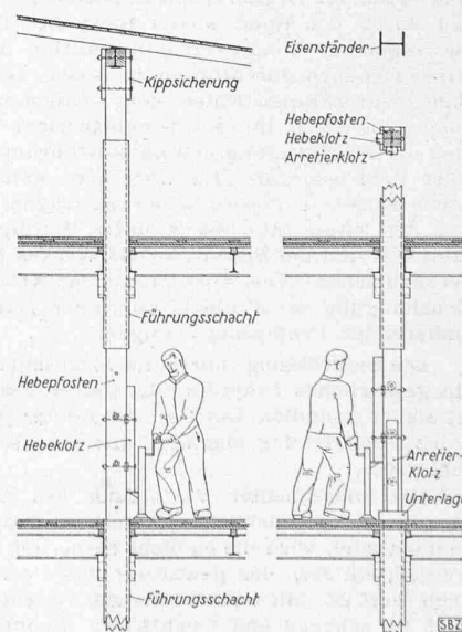
Abb. 3. Einzelheiten der Hebevorrichtung bei einem innern Ständer, Masstab 1:80
