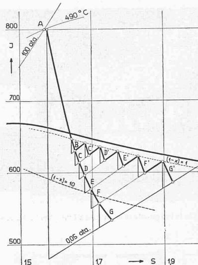
Abb. 1. Das J-S Diagramm einer Dampfturbine mit guter Entwässerung durch starke Umlenkung in der Gleichdruckschaufelung zeigt, dass die effektive Nässe (Linienzug A B' C' D' E' F' G') nur gering ist, während die theoretische Nässe (Linienzug A B C D E F G) bei Betrieb ohne Entwässerung 15% wäre
