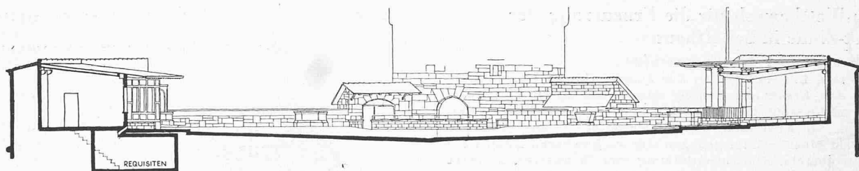
SCHNITT A-A
