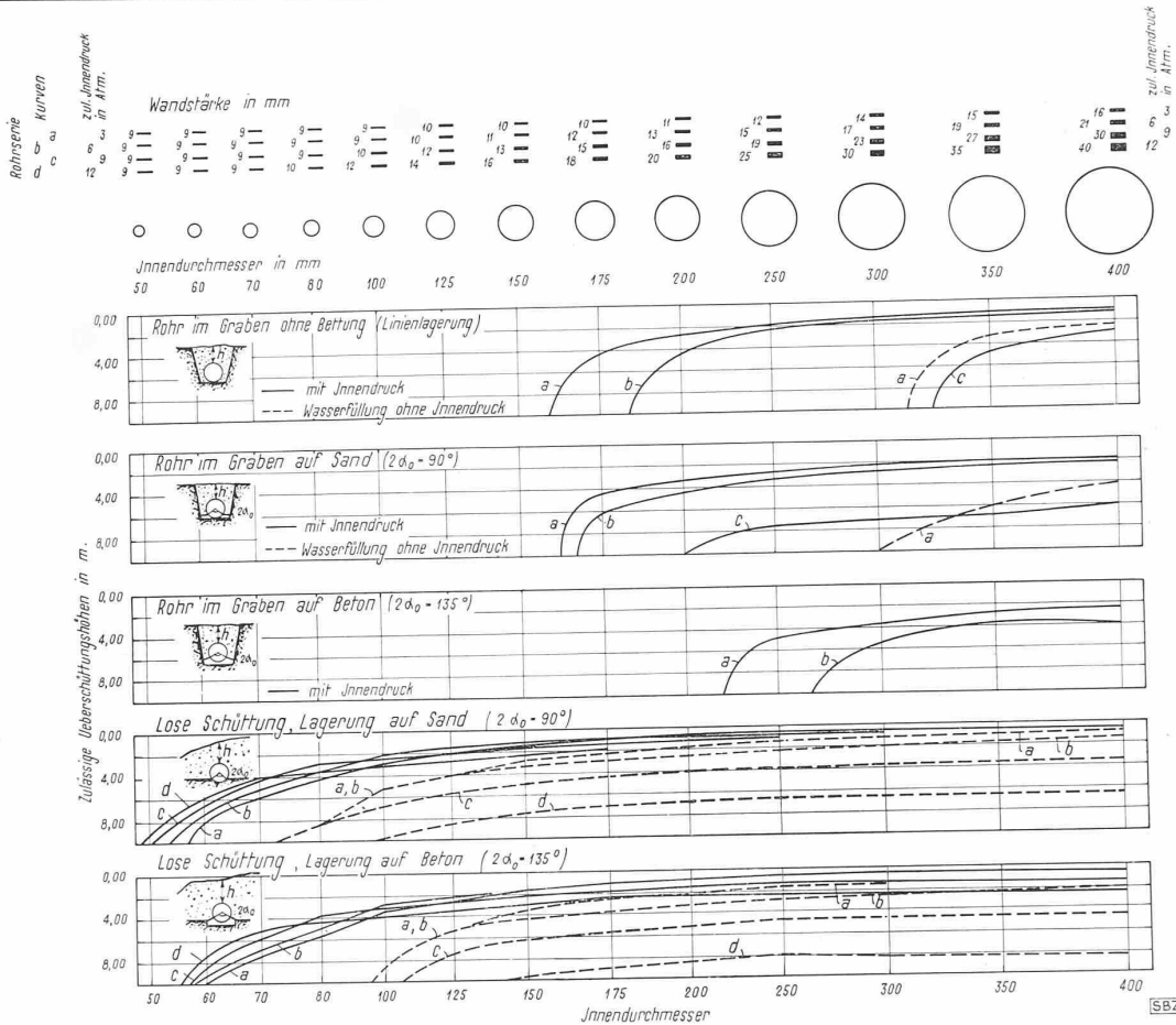
Abb. 21. Zulässige Verlegetiefen für stetig gelagerte Eternitröhren
