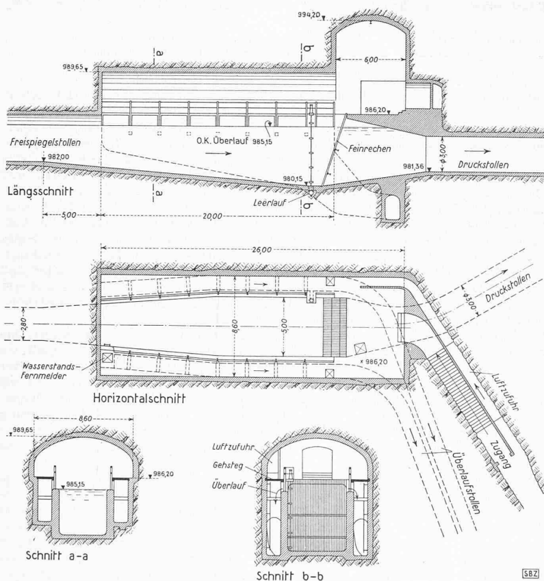
Abb. 16. Ueberlaufkammer bei Km. 6.86
