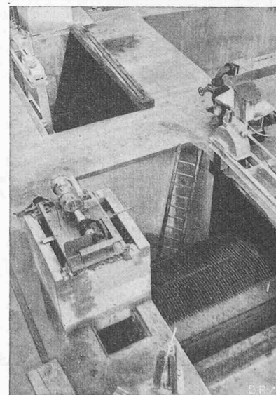
Abb. 6. Rotierender Trommelrechen
