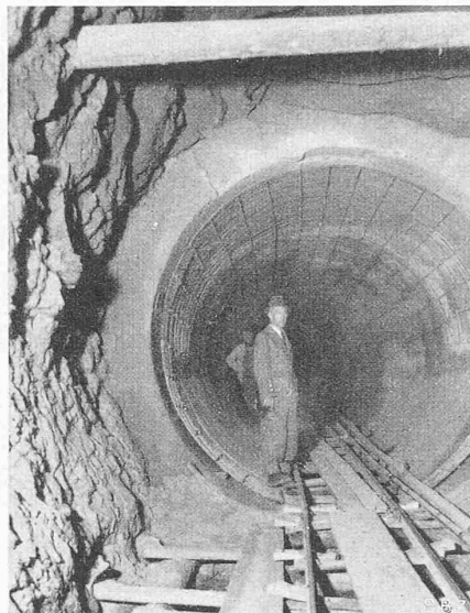
Abb. 13. Druckstollenprofil mit armierter Gunitauskleidung
