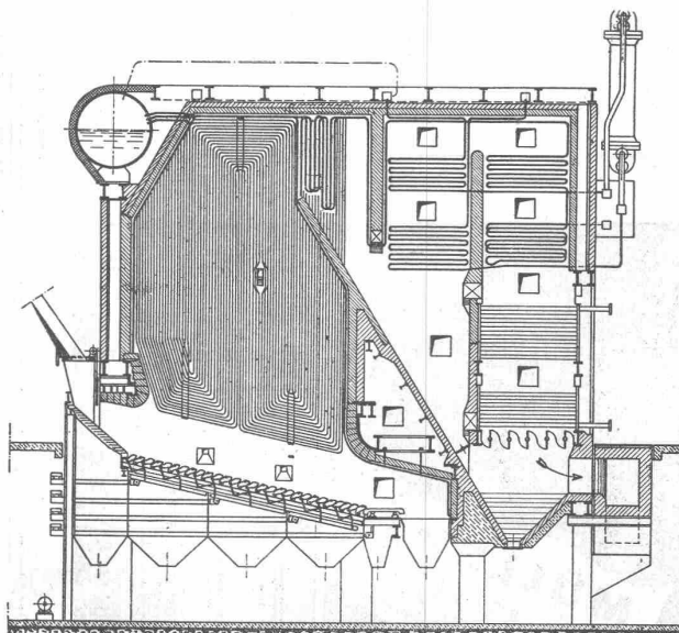
BUSS-La Mont-Dampferzeuger für 32/40 t/h, 50 at, 460° C, ausgerüstet mit BUSS-ÜBERSCHUBROST .
