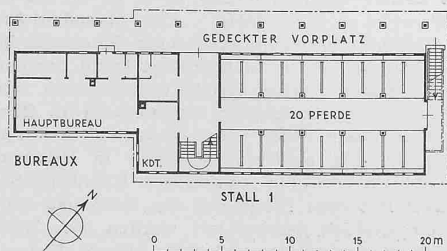
Abb. 1. Grundriss 1:500 einer militärischen Pferdekuranstalt, Ställe 1, 2 und 3
