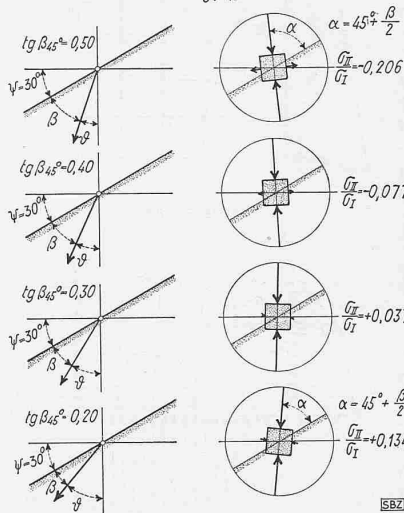
Abb. 4a. Metamorphe Spannungsänderung der geneigten Schneedecke beim Verdichtungs- bzw. Kriechvorgang. Die verschiedenen Werte \lg \beta_{45^\circ} kennzeichnen die den aufeinanderfolgenden Stadien der Verdichtung entspr. Kriechwinkel \beta für \psi=45^\circ [6]
