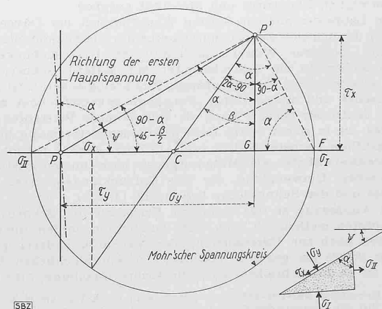
Abb. 3a. Konstruktion der Hauptspannungen in einem Punkte P der geneigten plastischen Schicht (dreieckförmiges Kriechprofil)
