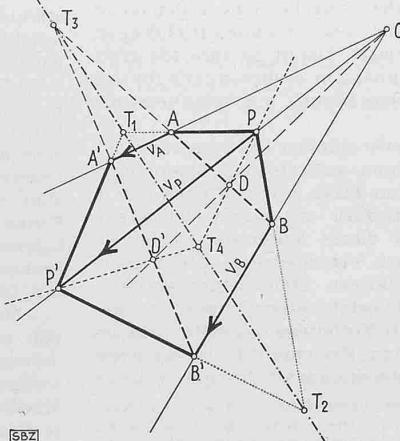
Abb. 5a. Zentrale Kollineation. C = Zentrum, T_1 - T_2 = Axe der zentr. Kollineation
