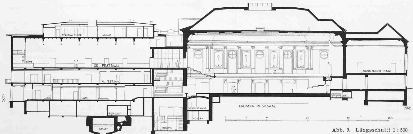
Abb. 9. Längsschnitt 1:500
