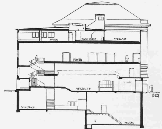
Abb. 11. Schnitt durch den Vestibule-Trakt. — 1:500
