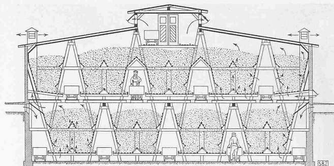
Abb. 2. Zweistöckiges Kartoffellager, System Karch, 1 : 200
