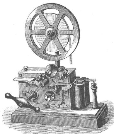
Alter Morse-Farbschreiber
