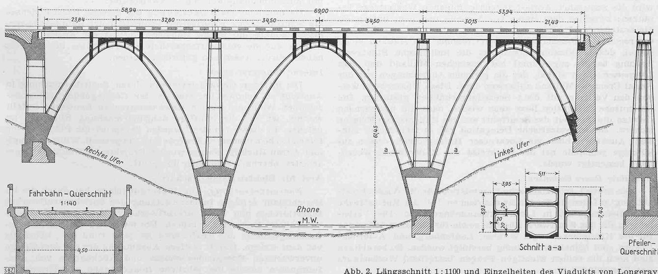
Abb. 2. Längsschnitt 1:1100 und Einzelheiten des Viadukts von Longerau
