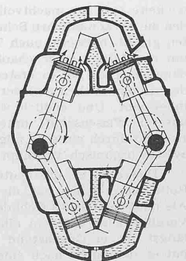
Abb. 9. Doppelkurbelwellenmotor mit abgeknickten Zylindern, Patent Saurer
