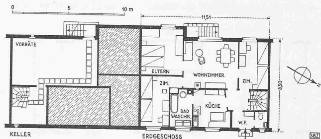
Abb. 3. Eingeschossige 4-Z.-Häuser (Typ 4/1) der 12. Etappe. 1:800
