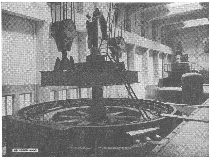
Der Rotor eines der Verbois-Grossgeneratoren wird montiert. Radstern, Radkranz und Pole sind gut sichtbar
