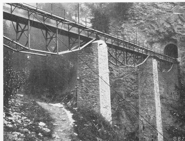
Abb. 20. Der umgebaute Viadukt mit drei einfachen Blechbalken
