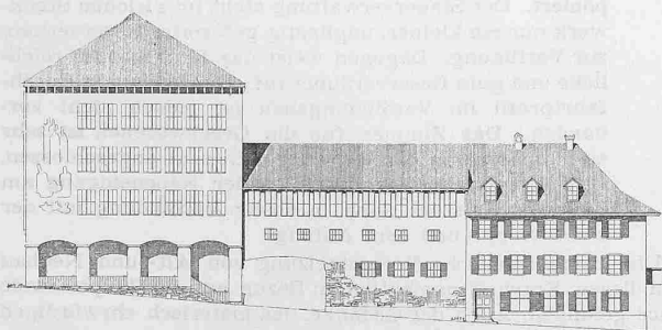
Nordostfront (Zollrain) und Nordwestfront (Halde) 1:600
