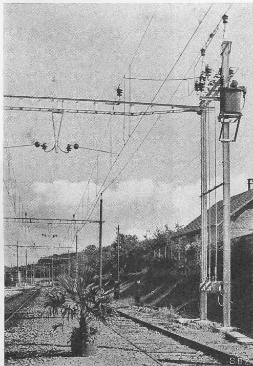
Abb. 1. Hörnerschaltposten mit Transformator
