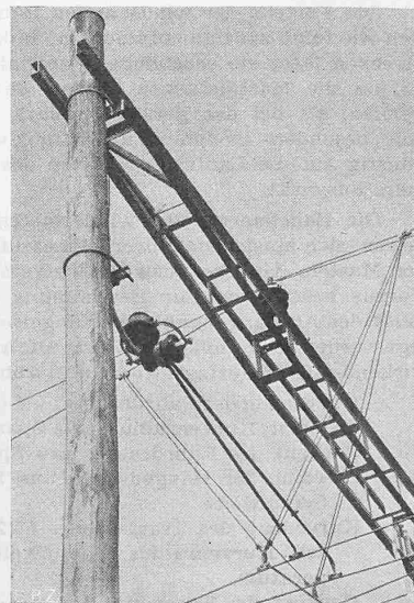
Abb. 4. (oben) Gleistrenner
