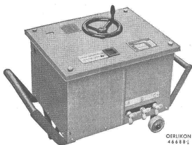
Schweisstransformator Typ EST-K 175 für max. 175 A, mit stufenloser Schweisstrom-Regulierung
