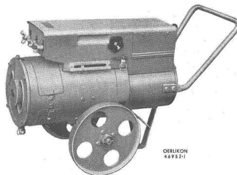
Schweissgruppe für max. 230 A
