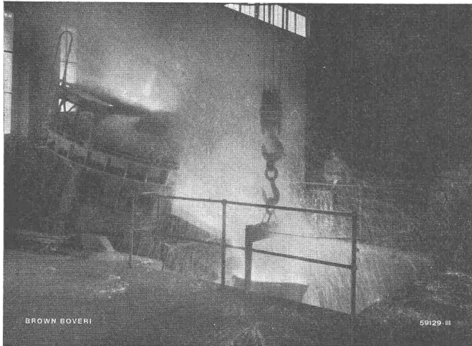
5-Tonnen Elektro-Schmelzofen in einem schweizerischen Stahlwerk beim Ausgiessen
