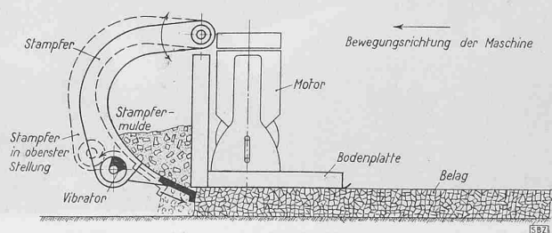
Abb. 2. Systemskizze des Strassenfertigerges Raco-Waldvogel
