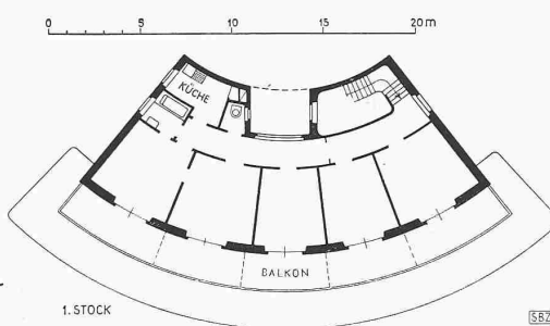
Abb. 17 u. 18. Grundrisse 1 : 400. — Die Zimmer im 1. Stock können einzeln oder als Apartement vermietet werden
