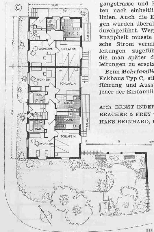
Abb. 5. Erdgeschoss-Grundriss Typ C. — 1:300
