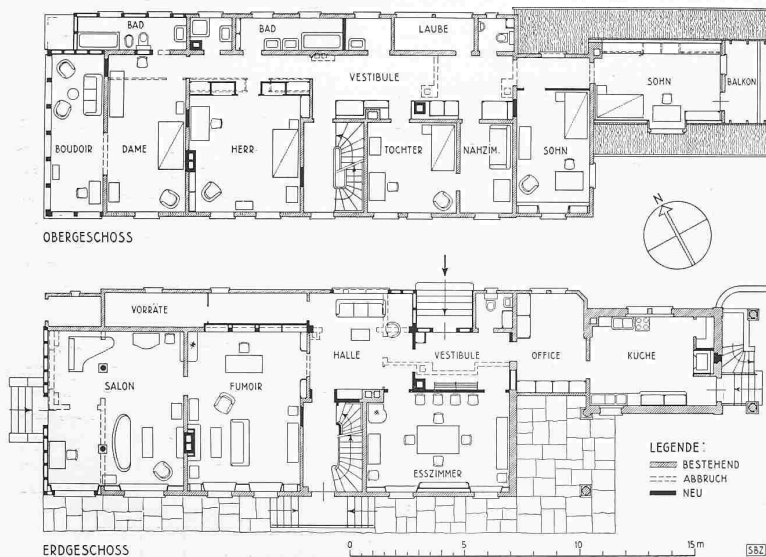
Abb. 5. Grundrisse, Masstab 1 : 300
