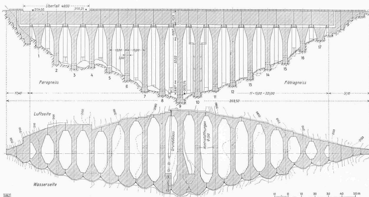
Abb. 1. Staumauer Lucendro. Längsschnitt und Grundriss. Masstab 1 : 1500. Text Seite 52
