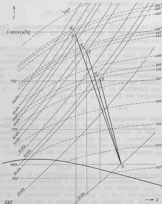
Abb. 4. Entropiediagramm mit den der Berechnung zu Grunde gelegten Zustandänderungen des Dampfes in der Gegendruck-Dampfturbine. d Zustand nach Ueberhitzer, g Zustand vor Turbine, h Zustand im Abdampfzustand
