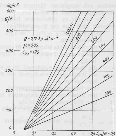
Abb. 26. Für den Start auf Hartbelagpiste zulässige Flächenbelastungen in Abhängigkeit des Schubfaktors bei gegebenen Rollstrecken
