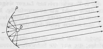
Abb. 3. Sehr kurze elektromagnetische Schwingungen werden wie Lichtwellen reflektiert. D Dipol, P Parabolspiegel
