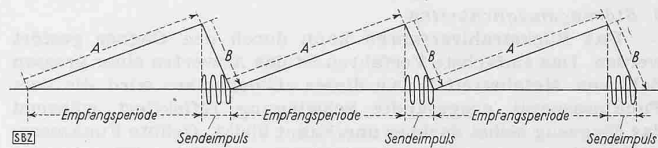
Abb. 10. Zeitlicher Verlauf des Sendens und Empfangens
