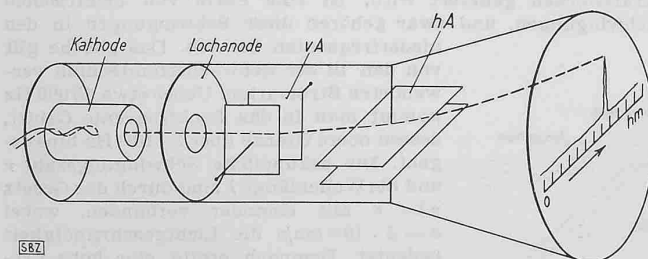
Abb. 11. Entfernungsanzeige durch den Elektronenstrom auf dem Schirm des Braunschens Rohrs. vA vertikale Ablenkplatten (Kondensatorwirkung), hA horizontale Ablenkplatten.
