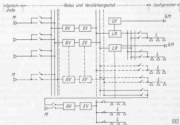
Abb. 1. Blockschema einer Lautsprecher-Grossanlage mit Sprechstellen, Verstärker- und Relais-Gestell, Lautsprecher-Gruppen und Nebenstelle. Legende im Text
