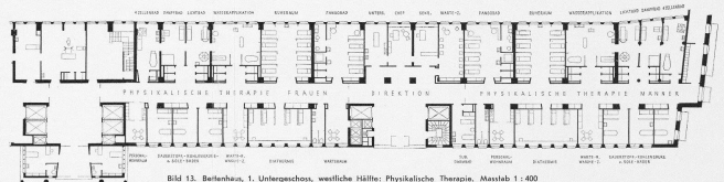
Bild 13. Bettenbau, 1. Untergeschoss, westliche Hälfte: Physikalische Therapie. Masstab 1:400
