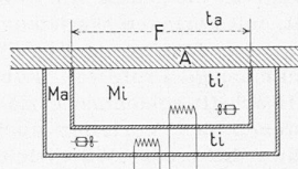
Bild 10. Messprinzip zur Bestimmung der Wärmedurchgangszahl. A zu prüfendes Wandstück, F Berührungsfläche, Mi innerer Messraum, Ma äusserer Messraum, ti Temperatur in den Messräumen, ta Aussen-temperatur
