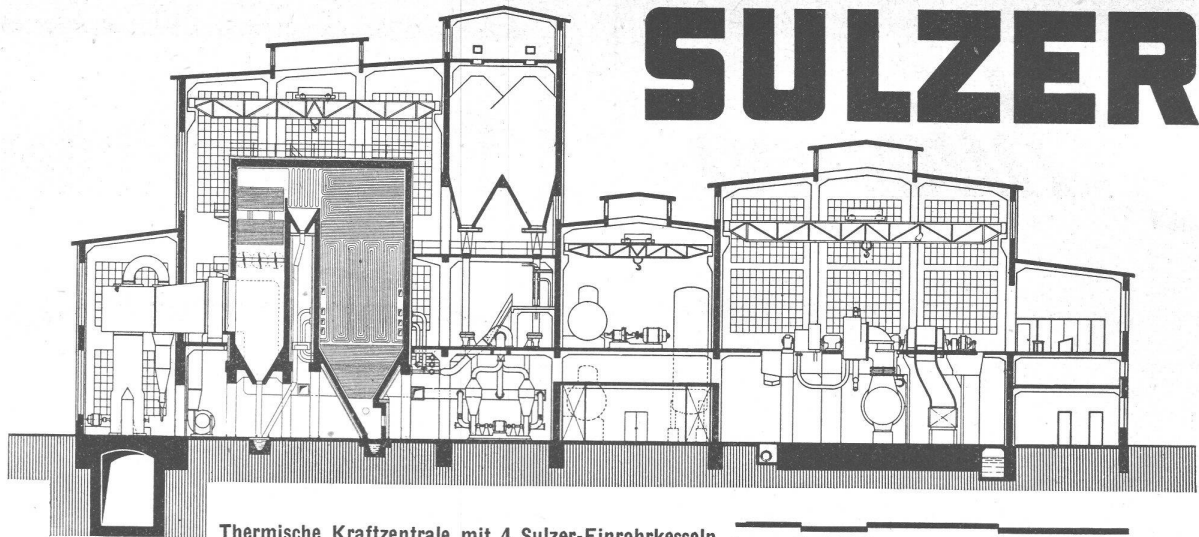
Thermische Kraftzentrale mit 4 Sulzer-Einrohrkesseln à 125 t/h, 80 atü, 500° C und 4 Turbogruppen à 25 000 kW
