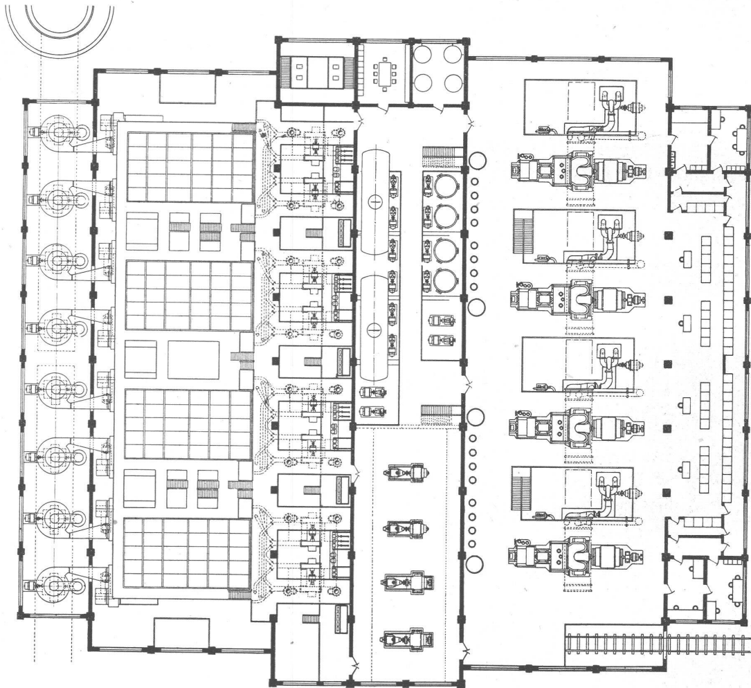
Thermische Kraftzentrale mit 4 Sulzer-Einrohrkesseln à 125 t/h, 80 atü, 500° C und 4 Turbogruppen à 25 000 kW
