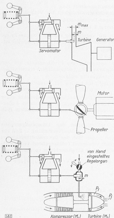
Bild 1 bis 3. Schematische Gegenüberstellung der Drehzahlregelung von Turbinen u. Flugzeug-Triebwerken
